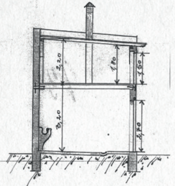
- SCHNITT E-F -
